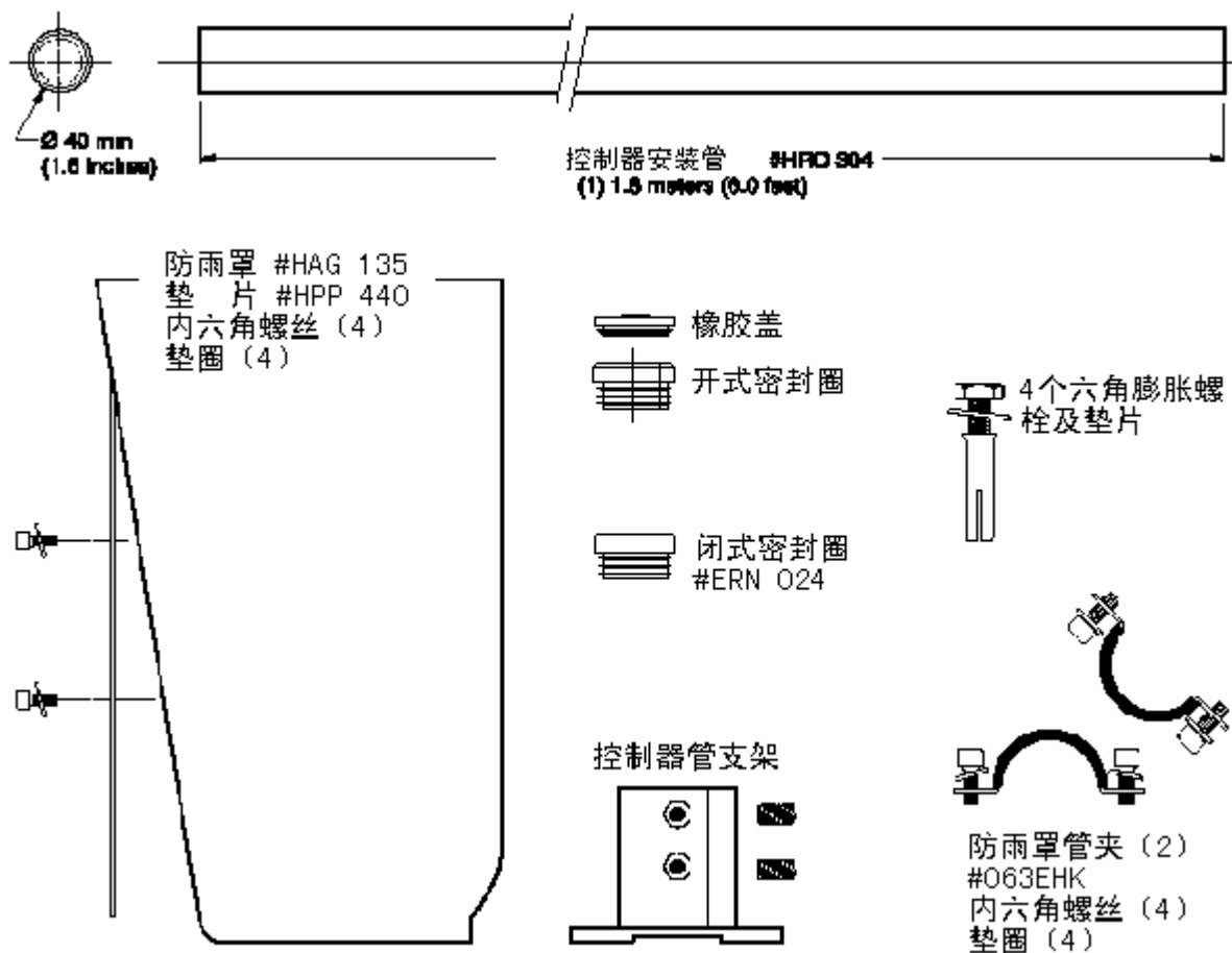
图1 控制器固定点安装附件（货号57344-00）
